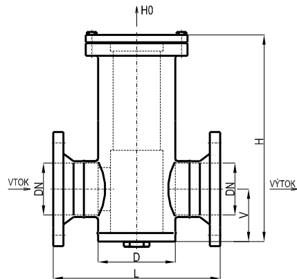
Rozměry a hmotnosti filtrů FU
