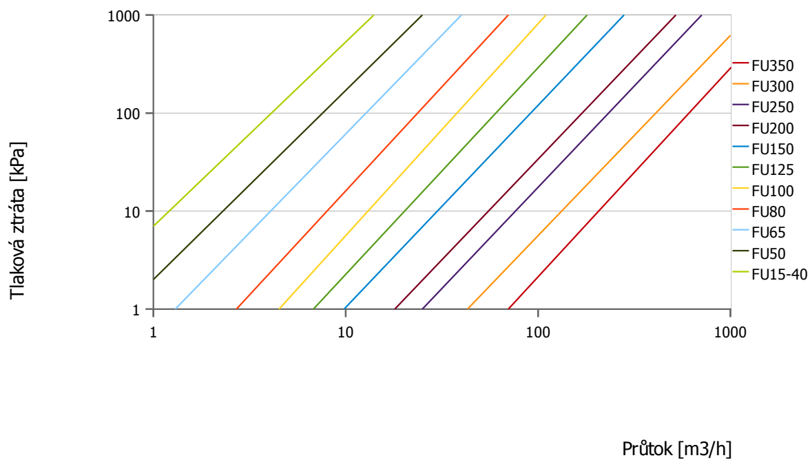
Tlakové ztráty filtrů FU s vložkou .x4
